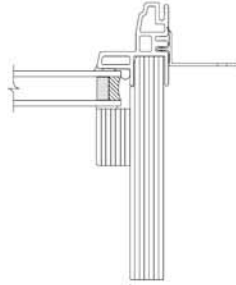
JAMB
